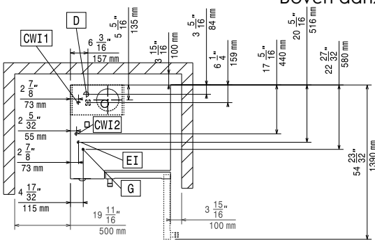
Boven aanzicht
